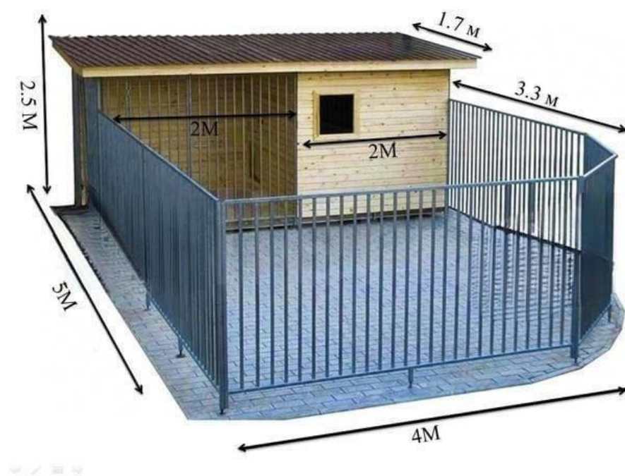
Рис. 2. Типовой проект вольера для служебных собак
