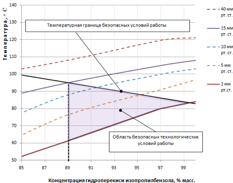
Рисунок. Зависимость температуры кипения ГП ИПБ от концентрации и остаточного давления
