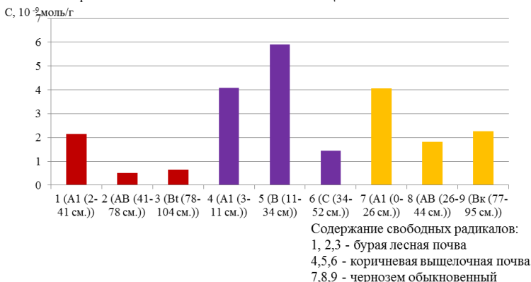
Рисунок. Содержание свободных радикалов в образцах почвы
